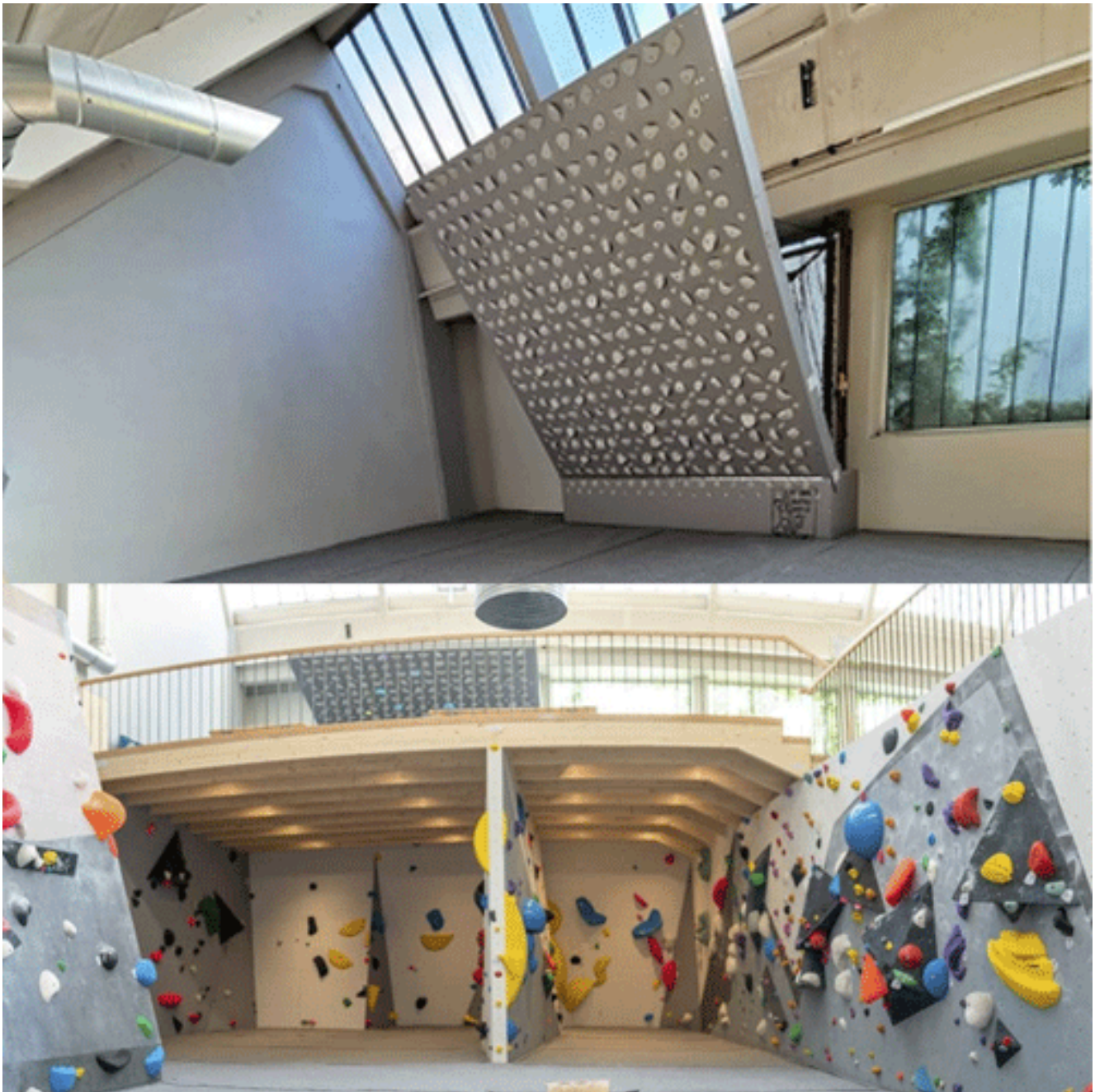
Abbildung 29: Umbau Blockfabrik Wien, ca. 120m 2 Boulderfläche mit 60m 2 Zwischenboden und elektrisch verstellbarem 3,66x3,66m Kilterboard, Winter 2021
