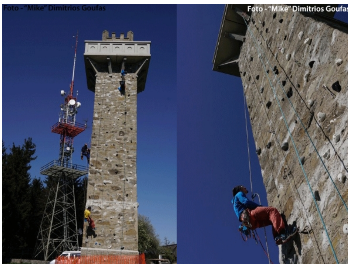
Abbildung 1, Adaption Elisabethwarte zum Klettern nach EN12572-1, ca. 162m 2 Kletterfläche, 15m Höhe, 2017, AV St.Peter/Au (LEADER Projekt)
